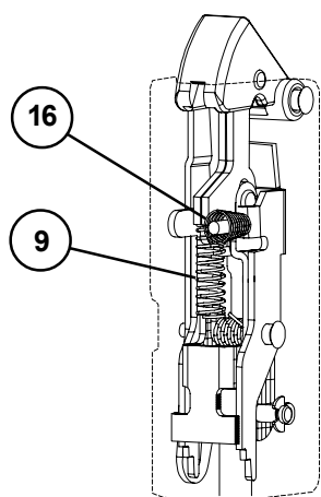
7547 Top Latch
